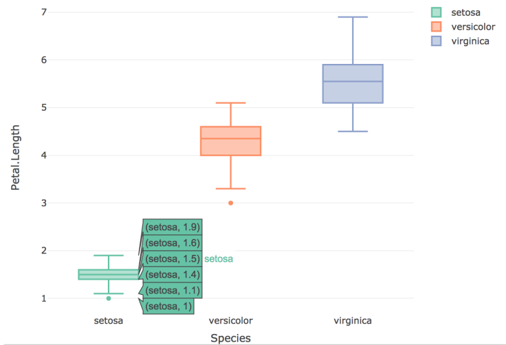
Figure 4: Diagrama de cajas o boxplot por especies con la librería plotly
